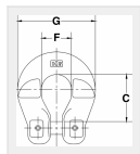
Plano de dimensiones
